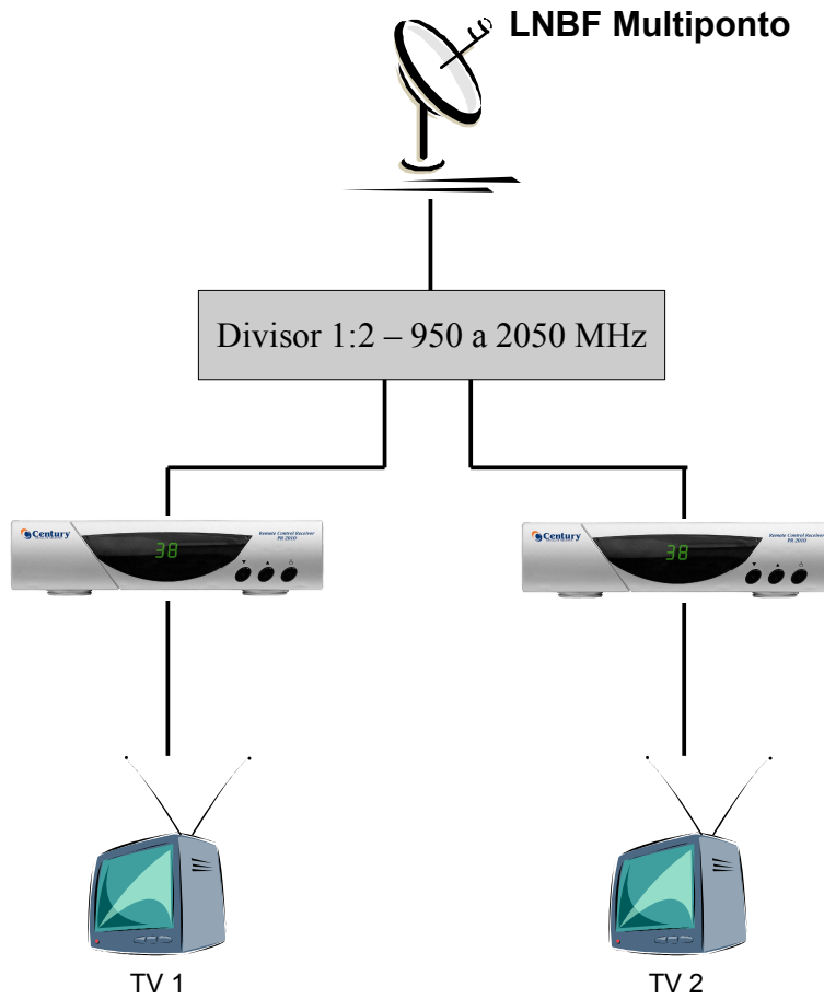
LIGAÇÃO DE 2 TV's EM UMA ÚNICA ANTENA
